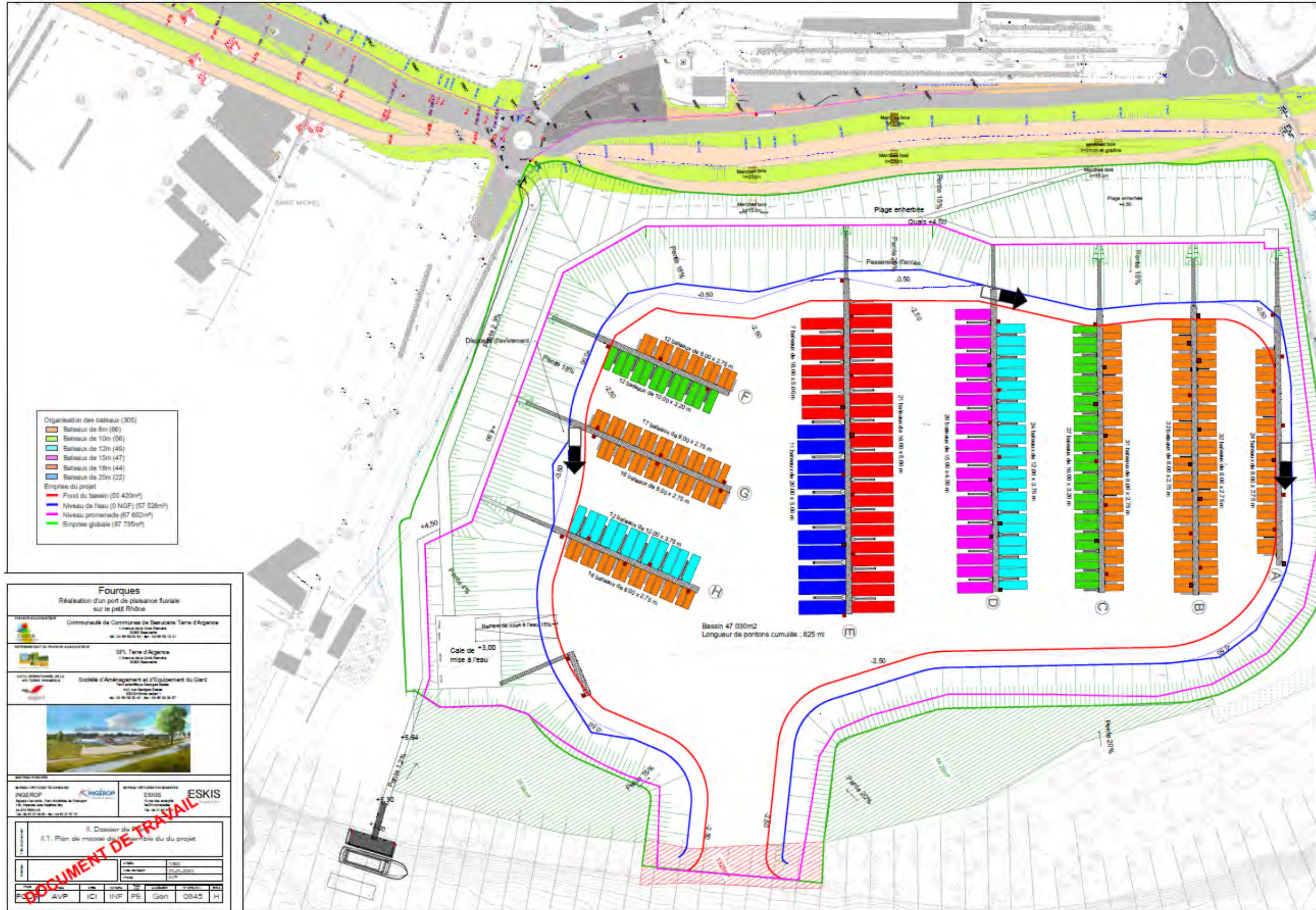
Figure 1 : Plan masse du port
